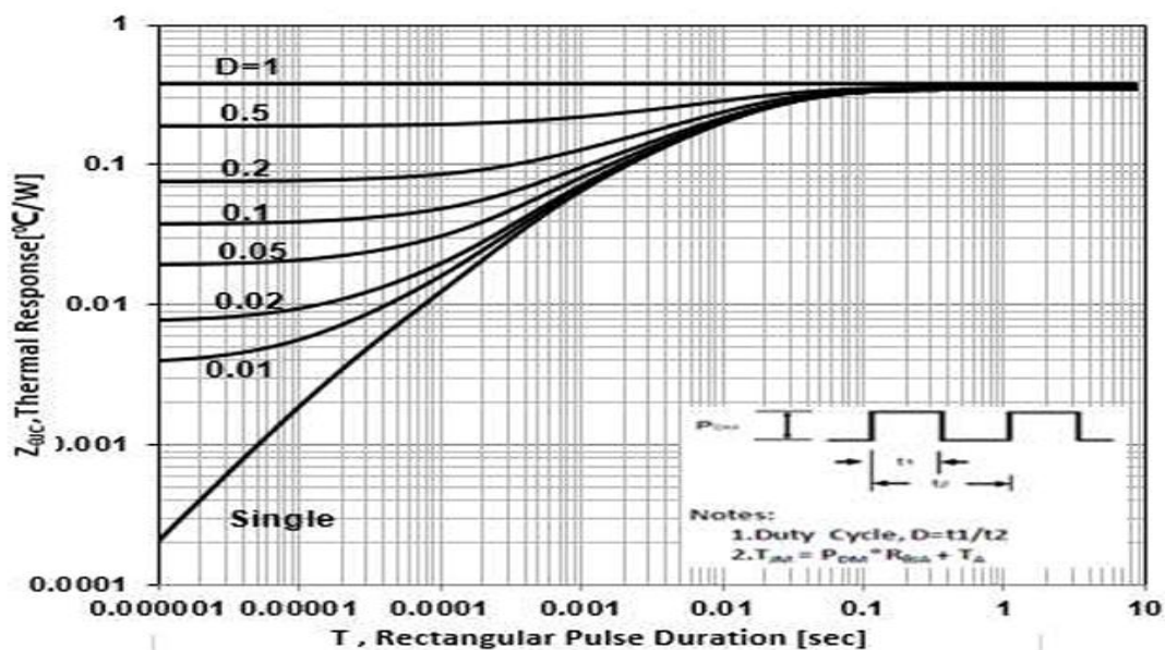
Fig 11 .Transient thermal impedance
