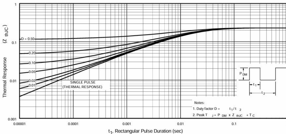
Fig 11 .Transient thermal impedance
