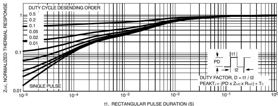
Fig 11 .Transient thermal impedance
