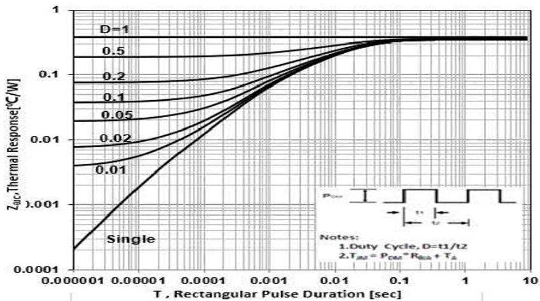
Fig 9 .Transient thermal impedance
