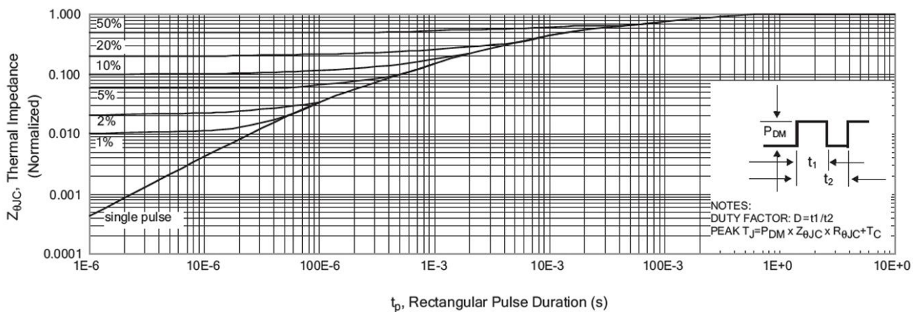
Fig 9 .Transient thermal impedance
