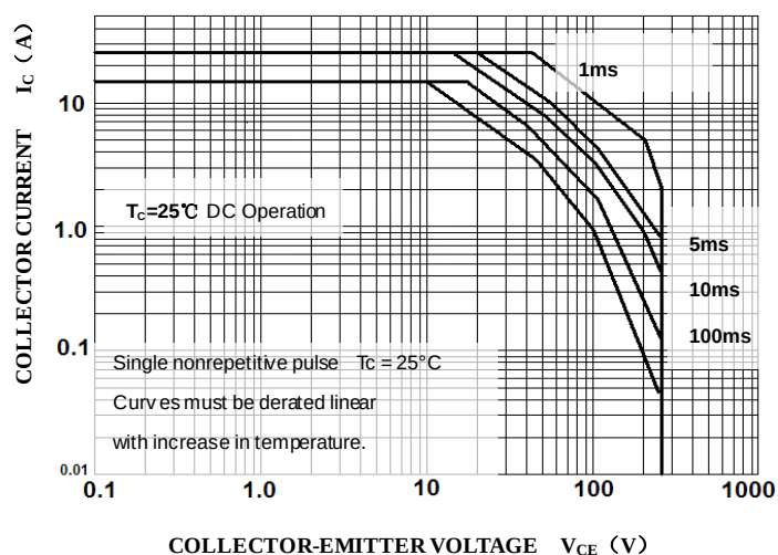
SOA
