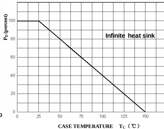
P_D - T_C
